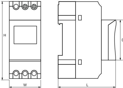
Размери (mm)
